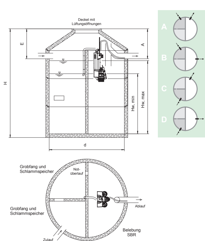
AQUAPRIMO® P Version Z = Kettenaufhängung
